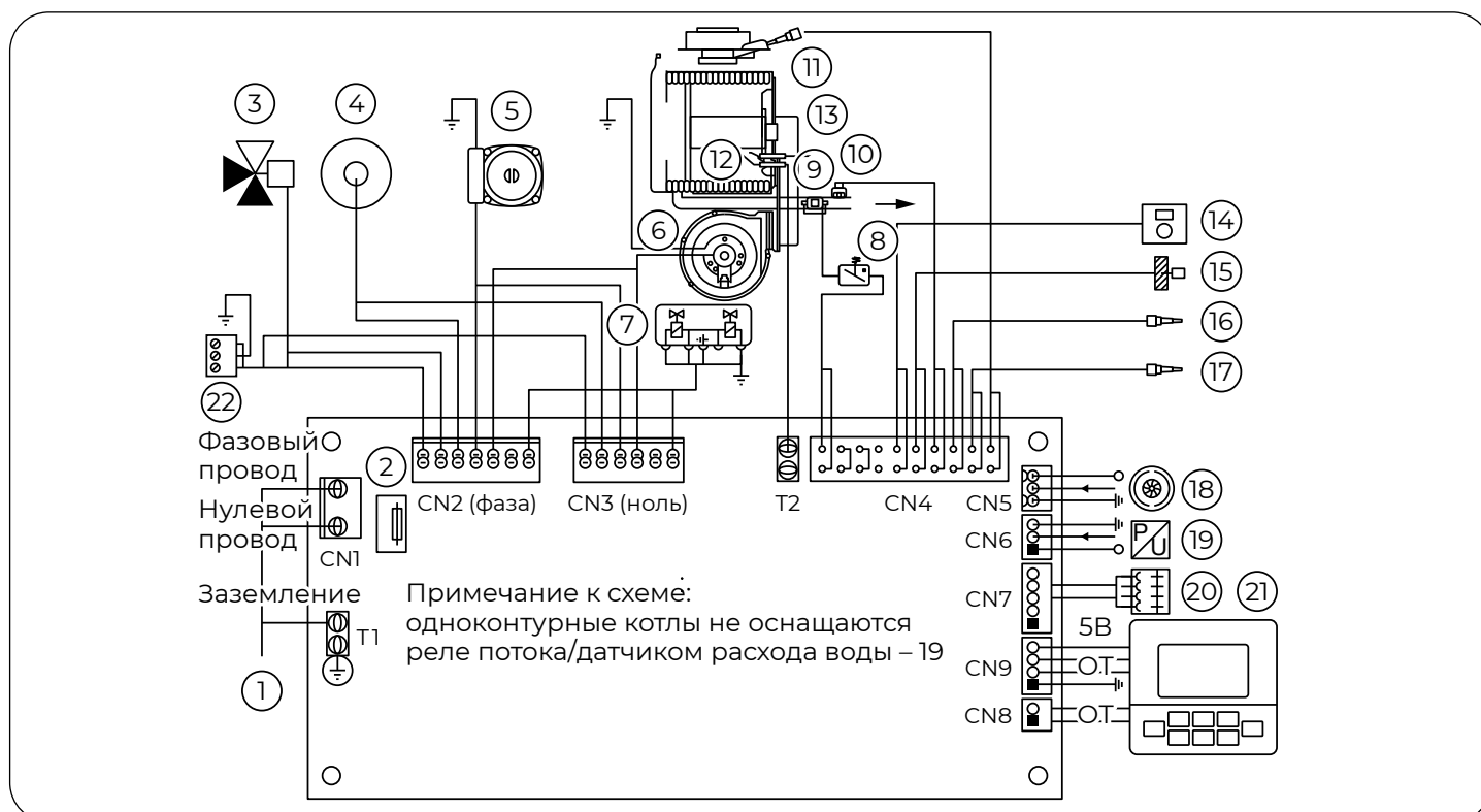
Рис. 35. Электрическая схема.
